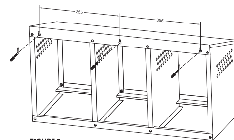
FIGURE 3 Marquer les trous de la surface de montage en utilisant la boîte de couvaion comme modèle.
