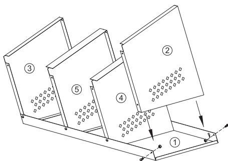
FIGURA 1 Instale los paneles terminales en los lados derecho e izquierdo y los dos paneles divisores como se ilustra y atornillelos
