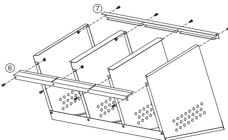
FIGURA 2 Coloque las crucetas frontal y posterior en los paneles como se ilustra y atornillelas
