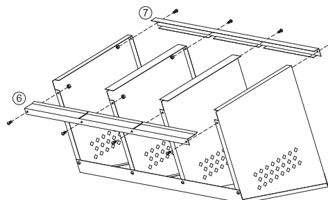
FIGURE 2 Ajuster les attelles transversales avant et arrière sur les panneaux, comme montré, et visser les vis.
