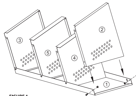
FIGURE 1 Installer les panneaux d'extrémité droit et gauche et les deux panneaux de division, comme montré, et visser les vis.
