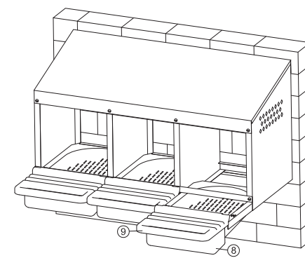
FIGURE 4 Suspendre les boîtes de couvaion en plastique et installer les couvercles de boîte de couvaion.
