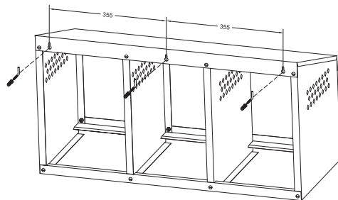
FIGURA 3 Marque los orificios en la superficie de montaje utilizando el nidal como plantilla
